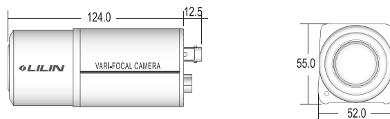
尺寸圖 單位：mm
