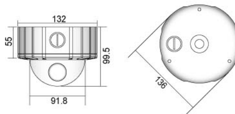
尺寸圖 單位：mm
